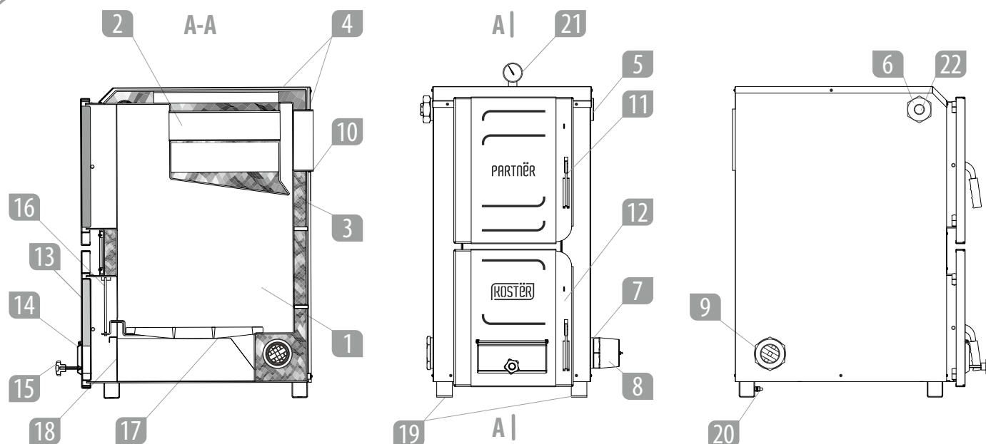
Рис. 1 Конструкция котла PARTNER
