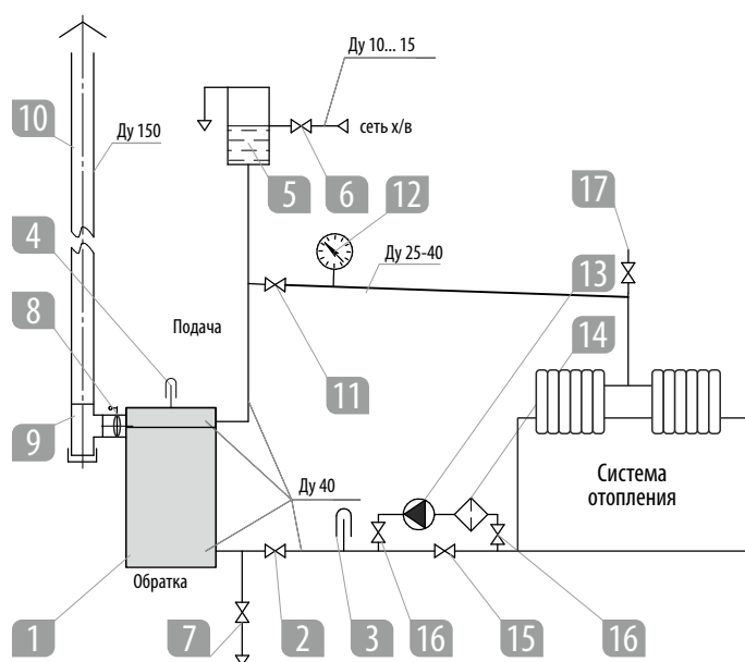
а) открытая система с принудительной циркуляцией
