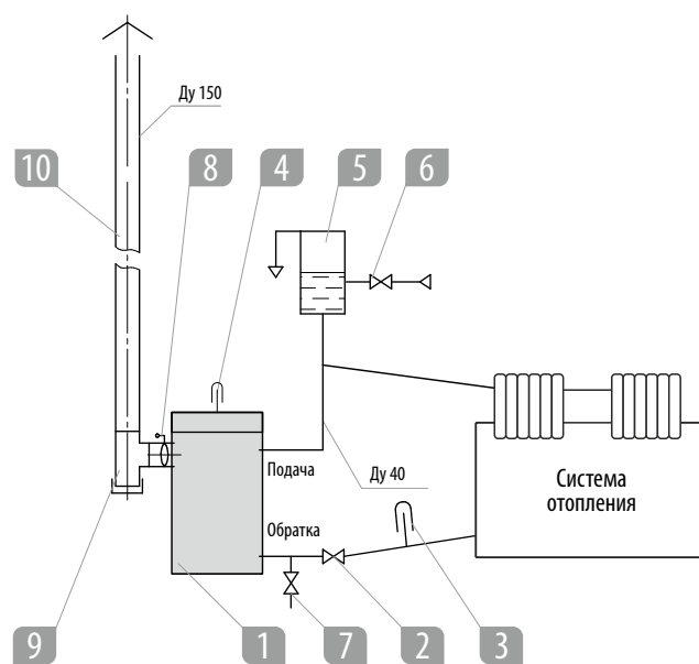
б) открытая система с самоточной циркуляцией
