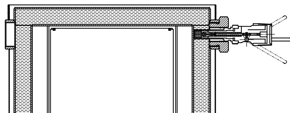
Рис.4 Установка регулятора горения
