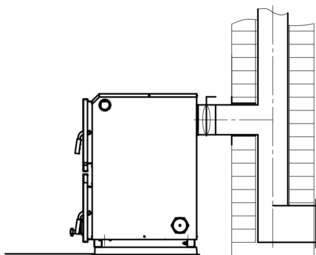
Рис. 7 Присоединение котла к кирпичному дымоходу при помощи вставленного стального дымохода.
