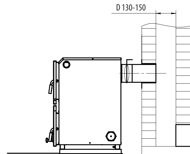
Рис.8 Присоединение котла к кирпичному дымоходу.
