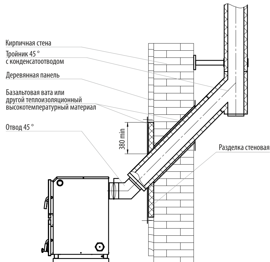
Рис. 5 Оптимальное присоединение котла к дымоходу расположенному за кирпичной стеной на улице.
