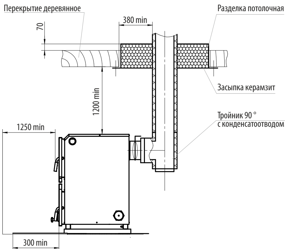
Рис. 9 Присоединение котла к дымоходу, проходящему через деревянное перекрытие.
