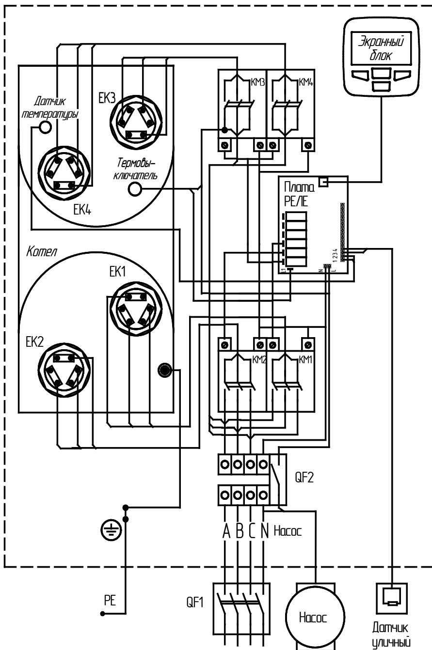
Рисунок 8. Схема подключения ЭВАH UNIVERSAL -60 - 14 -
