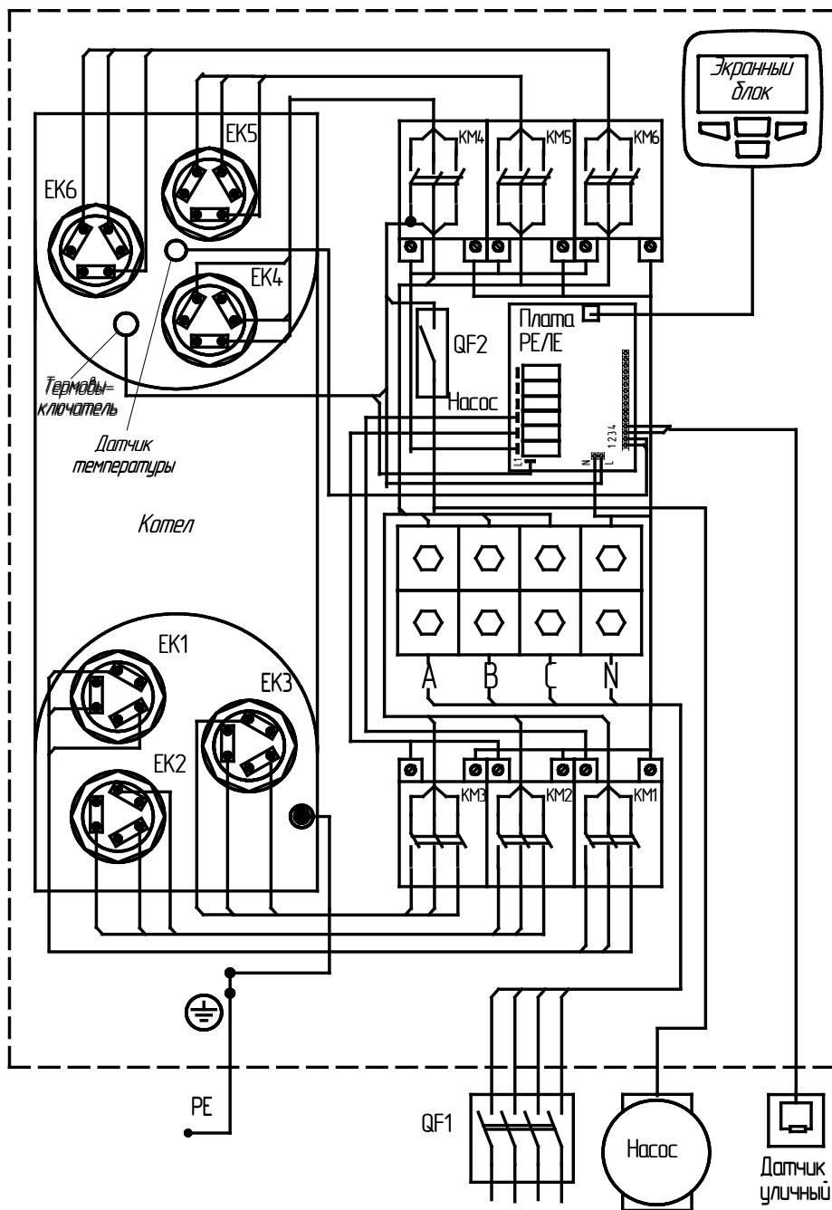
Рисунок 11. Схема подключения ЭВАГ UNIVERSAL -81, 96, 105, 120 - 17 -
